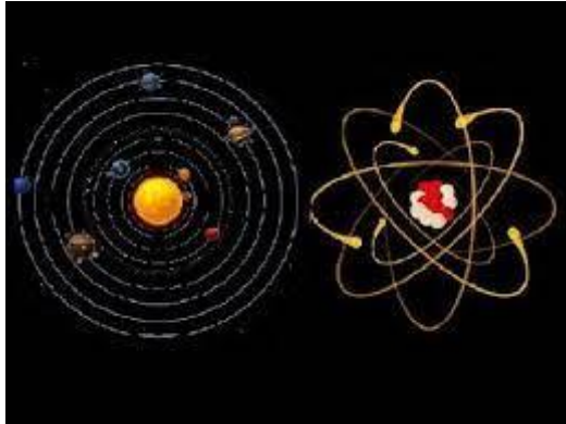
Sistema solar e um átomo
